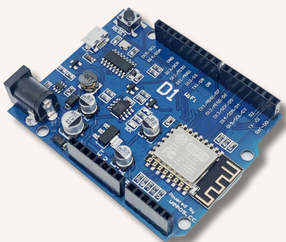
WeMos D1 R2 119฿
