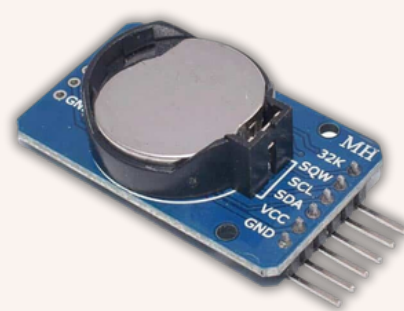
RTC Module 97฿
