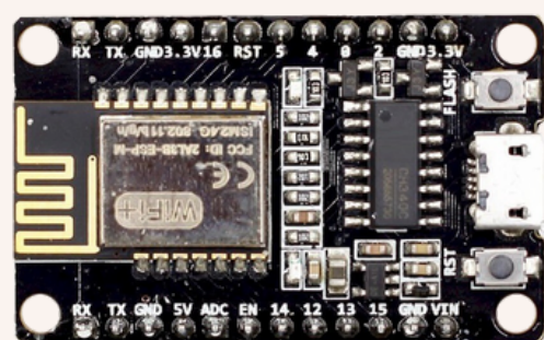
NodeMCU-M 149฿
