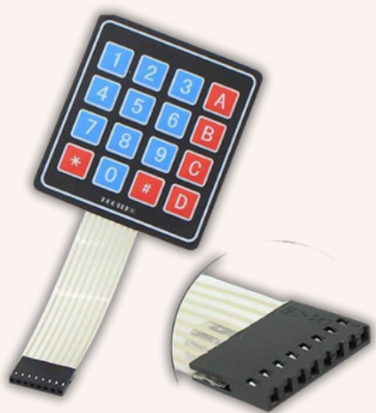
Keypad 4x4 25฿
